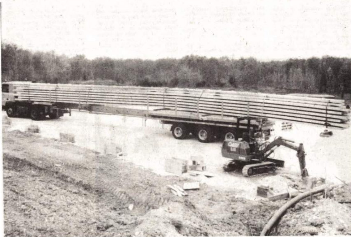
Les éléments de la charpente du manège sont arrivés, hier, à Darel. Il ne reste plus qu'à les assembler.
